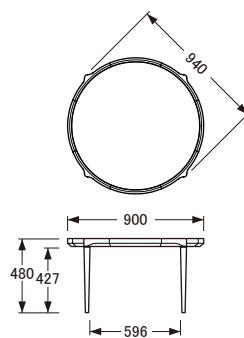
[90φ×H48]
