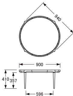
[90φ×H41]
