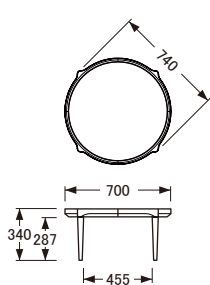
[70φ×H34]
