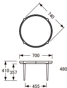
[70φ×H41]
