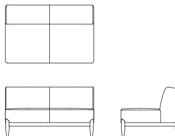
肘無ワイド2Pソファ L08440F OIL WN 【W/1260 D/830 H/720 SH/420】
