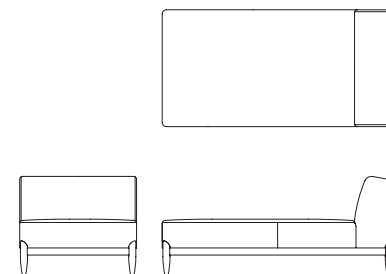
肘無シェーズロング L08430N OIL WN 【W/830 D/1630 H/720 SH/420】
