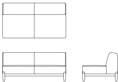
肘無3Pソファ L08440S OIL WN 【W/1490 D/830 H/720 SH/420】
